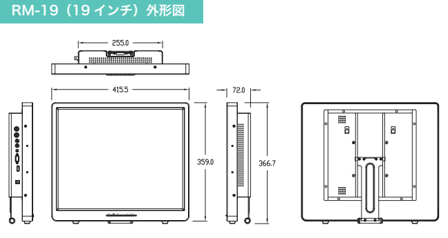
RM-19 (19 インチ) 外形図
