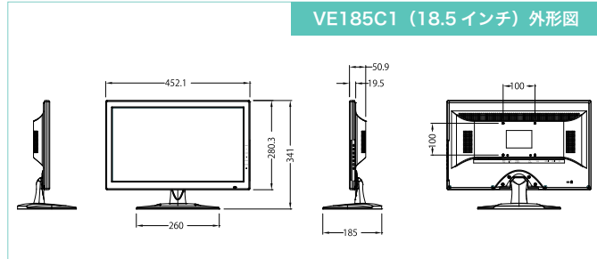
VE185C1 (18.5 インチ) 外形図
