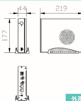
外形図
